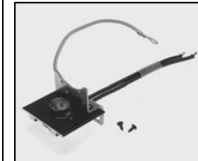
L4.79373.E Lampholder + lamp carriage Lampenfassung + Fassungsträger B 15 d 120V
