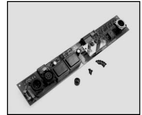
L4.84129.E DMX converter 230 V DMX Signalkonverter 230 V
