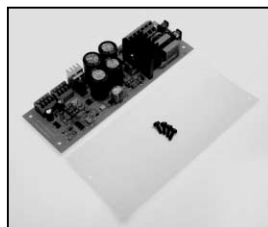
L4.84131.E Phase converter 120 - 230 V Phase Signalkonverter 120-230V
