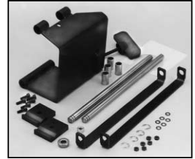
L4.83285.E Justable stirrup bracket set right Schwerpunktverstellung rechts
