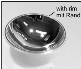
L4.80112.E New glass reflector from ser.no. 1258 (does not fit into reflectorholder to ser.no.363 - in this case please order L4.81179.E) Neuer Glasreflektor ab Ser. Nr. 1258 (passt nicht in Reflektorhalter bis Ser.Nr. 363 - in diesem Fall bitte L4.81179.E bestellen)
