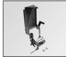
L4.83320.E Lampholder & carriage (lampheads to ser.no.1258 also need new reflector L4.80112.E) Lampenfassung & Fokusschlitten (Schweinwerfer bis Ser.Nr.1258 benö- tigen den neuen Reflektor L4.80112.E)
