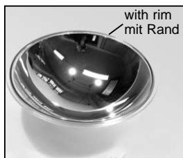
L4.80112.E New glass reflector from ser.no. 364 (does not fit into reflectorholder to ser.no.363 - in this case please order L4.80769.E) Neuer Glasreflektor ab Ser. Nr. 364 (passt nicht in Reflektorhalter bis Ser.Nr. 363 - in diesem Fall bitte L4.80769.E bestellen)
