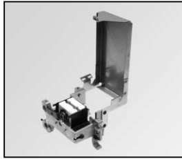
L4.83122.E Lamp holder+lamp carriage from ser.no. 4972, for earlier versions please order additionally L4.80062.E New glass reflector! Lampenfassung + Fokusschlitten ab Ser.Nr. 4972, für frühere Versionen bestellen sie bitte zusätzlich L4.80062.E Neuer Glasreflektor
