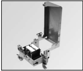
L4.83122.E Lampholder + lamp carriage Lampenfassung und Fokusschlitten
