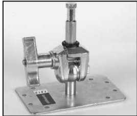
L2.84542.0 Holding plate with ball joint, stud 16mm Discontinued! Halteplatte mit Kugelgelenk, Zapfen 16mm Nicht mehr verfügbar!
