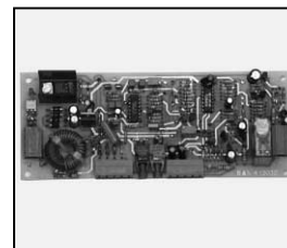
L4.82571.E Control board act. line filter Regelkarte akt. Netzfilter
