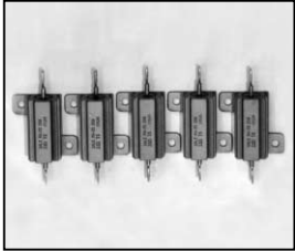
L4.82578.E Ignitor and start resistor-set (5 pieces) Zünd- und Startwiderstand-Set (5 Stück)
