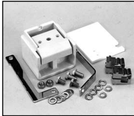
L4.79117.E Lampholder cpl. (repair only according to manufacturing instruction and with genuine gages) Lampenfassung kpl. (Reparatur nur nach Fertigungsvorgabe und mit original Einstell-Lehren)
