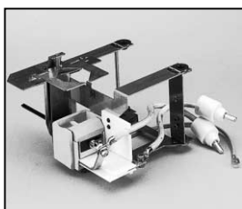
L4.79123.E Lamp holder + lampholder (repair only according to Manufacturing Instruction and with genuine gages) Lampenfassung und Fassungsträger (Reparatur nur nach Fertigungsvorgabe und mit original Einstell- Lehren)
