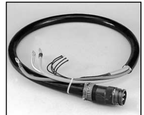
L4.79115.E Mains cable Scheinwerferkabel
