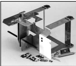
L4.79116.E Lamp carriage (repair only according to Manufacturing Instruction and with genuine gages) Fassungsträger (Reparatur nur nach Fertigungsvorgabe und mit original Einstell- Lehren)
