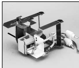
L4.79123.E Lampholder + lampholder (repair only according to Manufacturing Instruction and with genuine gages) Lampenfassung und Fassungsträger (Reparatur nur nach Fertigungsvorgabe und mit original Einstell- Lehren)
