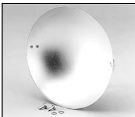
L4.71857.E Reflector Reflektor
