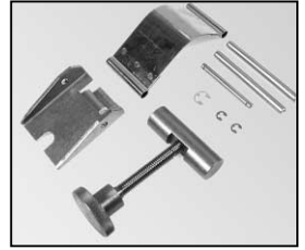
L4.71055.E Mounting set for lamp to ser.no.661 Befestigungs-Set für Lampe bis Ser.Nr.661
