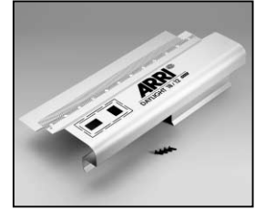
L4.71165.E Internal side baffle right Mantelstromblech rechts
