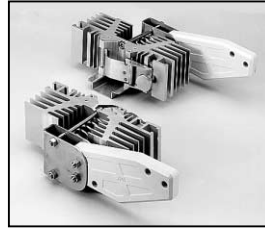
L4.71054.E Lampholder to ser.no.661 Lampenhalter bis Ser.Nr.661
