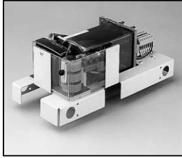
L4.71048.E Ignitor Zündgerät
