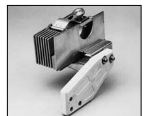
L4.71566.E f. x 25,4 Lamp holder left high voltage Lampenhalter links 380 V Ausführung
