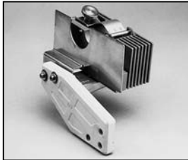
L4.71737.E f. x 30,0 Lamp holder right low voltage Lampenhalter rechts 220–240 V Ausführung
