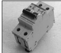
L4.75728.E (BCA 6000) Magnetothermal protection Sicherungsschalter
