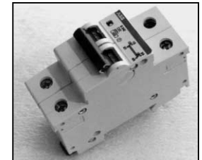
L4.75725.E (BCA 4000-3) Magnetothermal protection 380 V Sicherungsschalter 380 V
