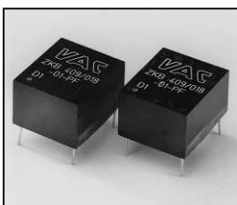
L4.82383.E Ignition Transformer (2 pieces) Zündübertrager (2 Stück) (ADM 20)
